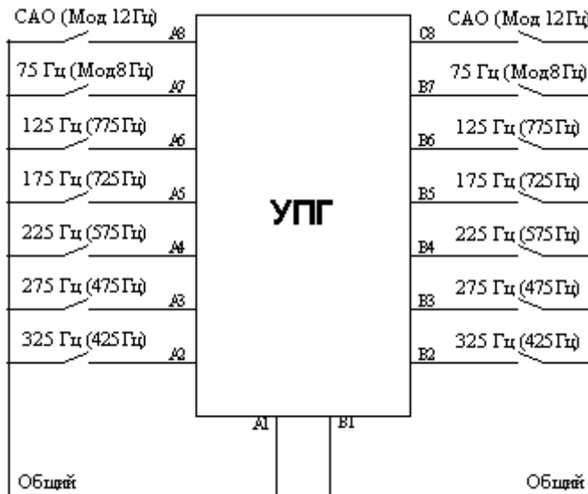
Схема частотоподающих переключателей для УПП-2
